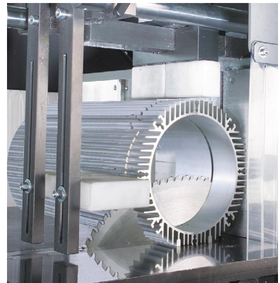
Profilspanneinrichtung
